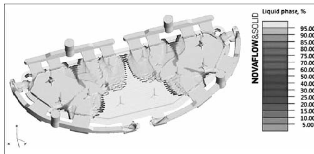
■ 1. ábra. A beömlőrendszer kialakítása és a formatöltés szimulációja 4 szekciós beömlőrendszerrel, a képen a folyékony fázis aránya 75% feltöltési hányadnál
