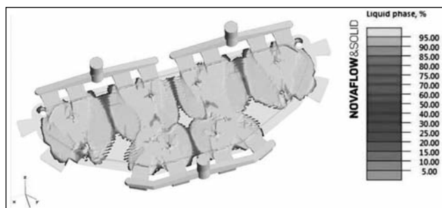
■ 2. ábra. A beömlőrendszer kialakítása és a formatöltés szimulációja 3 szekciós beömlőrendszerrel, a képen a folyékony fázis aránya 70% feltöltési hányadnál
