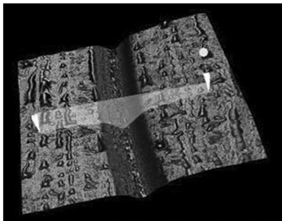
10. ábra. A 2 MHz ismétlési frekvenciájú, 30 \mu\text{J} impulzusenergiájú lézersugárral készült szublimációs árok fénymikroszkópi képe
