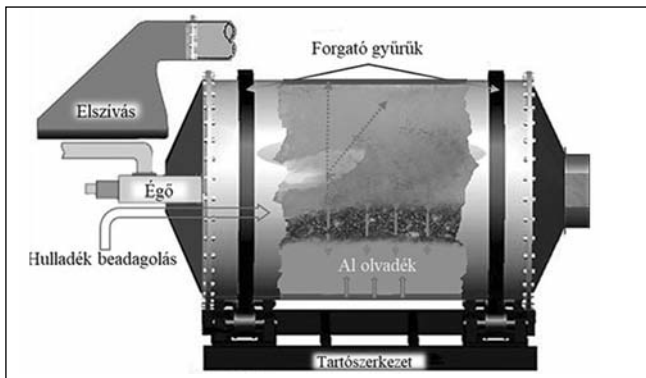
■ 4. ábra. Fekvő forgódobos kemence
