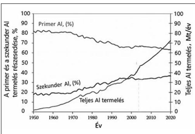
■ 1. ábra. A primer és szekunder fém megoszlása a teljes termelésben [4]
