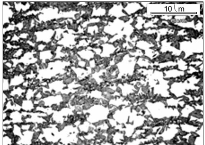
Kettős fázisú, DP-acél optikai mikroszkópi képe ferritmátrixba ágyazott martenzitszigetekkel
