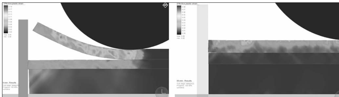
■ 11. ábra. A többrétegű termékek melegen hengerlésének végeselemes modellje
