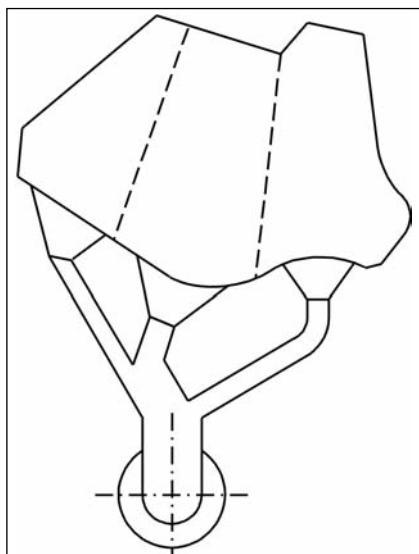
■ 8. ábra. A formaüreg részekre osztása
