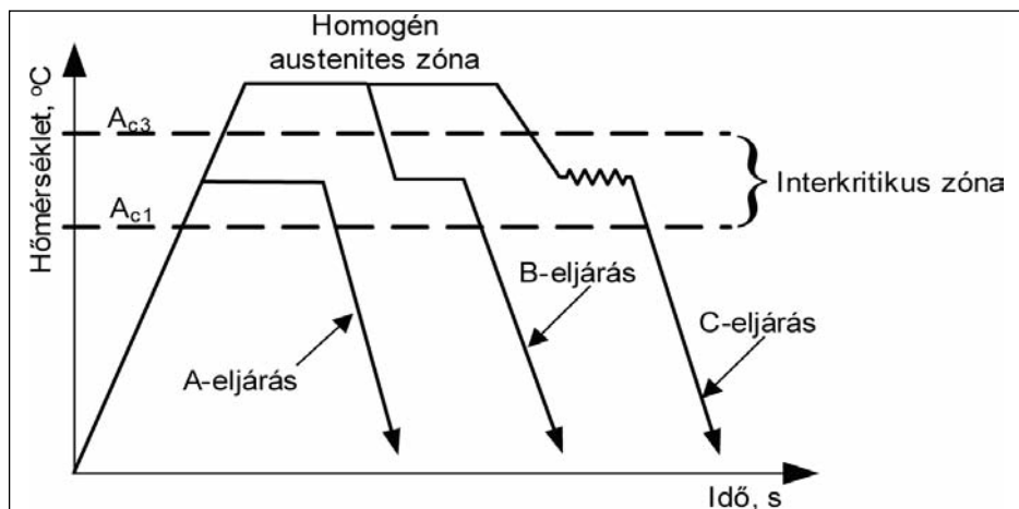
■ 5. ábra. DP-acélok különböző gyártási lehetőségeinek sematikus hőmérséklet-ido diagramja
