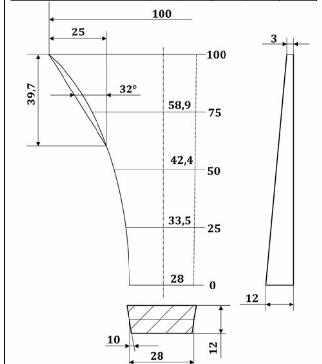
■ 10. ábra. A legyező alakú elosztó geometriai kialakítása
