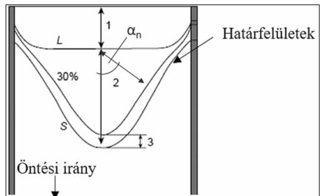
6. ábra. Az öntés közben kialakuló fázishatárok, zónák geometriája (L = likvidusz; S = szolidusz, és 30% szilárd fázist tartalmazó határfelület; (1 + 2 + 3) = olvadékot tartalmazó zónák) és az \alpha_n szög az öntött tuskó tengelye és a kristályosodási front normális iránya között [1, 6]
