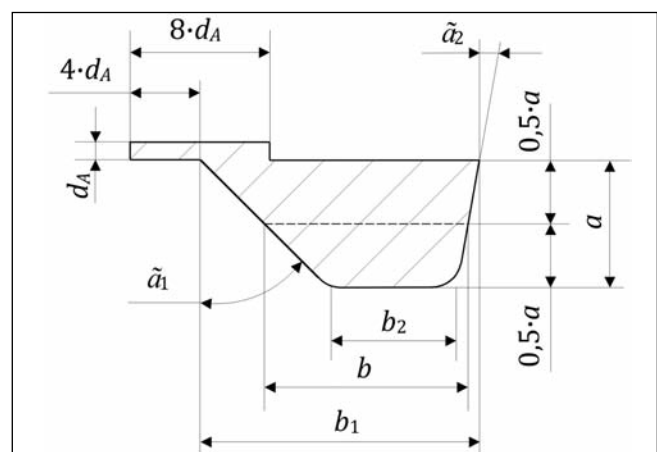
■ 11. ábra. A tangenciális alakú elosztó és a bekötőcsatorna metszetének méretviszonyai
