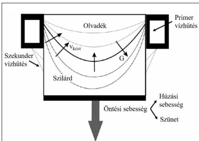
5. ábra. Az öntött tuskó kristályosodását érintő tényezők, ahol v_{\text{krist}} : a kristályosodás sebessége [mm/s] és G : a hőmérséklet-gradiens [ ^{\circ}\text{C}/\text{mm} ]. R. Nadella és társai [1] publikációja nyomán
