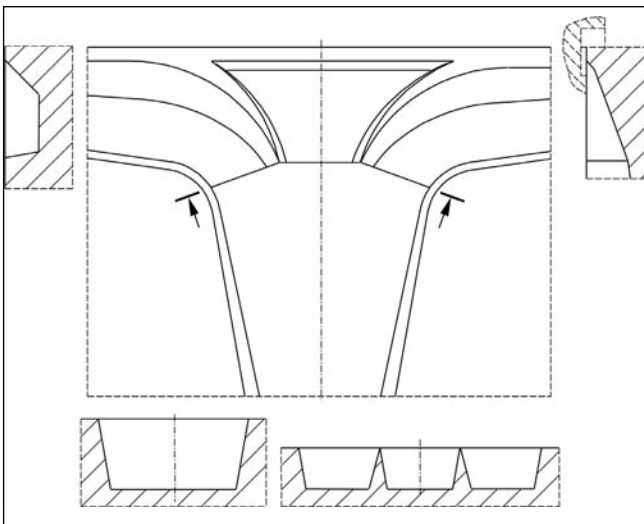
■ 14. ábra. A tangenciális alakú elosztó középső részének (deltaterület) kialakítása a szerszámotétben
