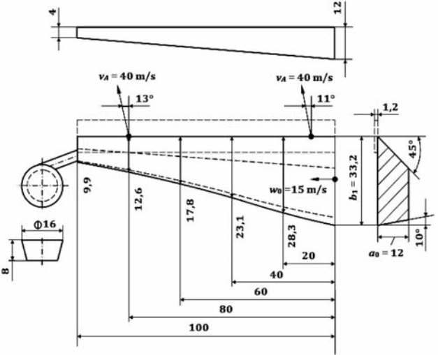
■ 16. ábra. Az egyenletesen szűkülő keresztmetszetű tangenciális elosztó vázlata és méretábrázolása
