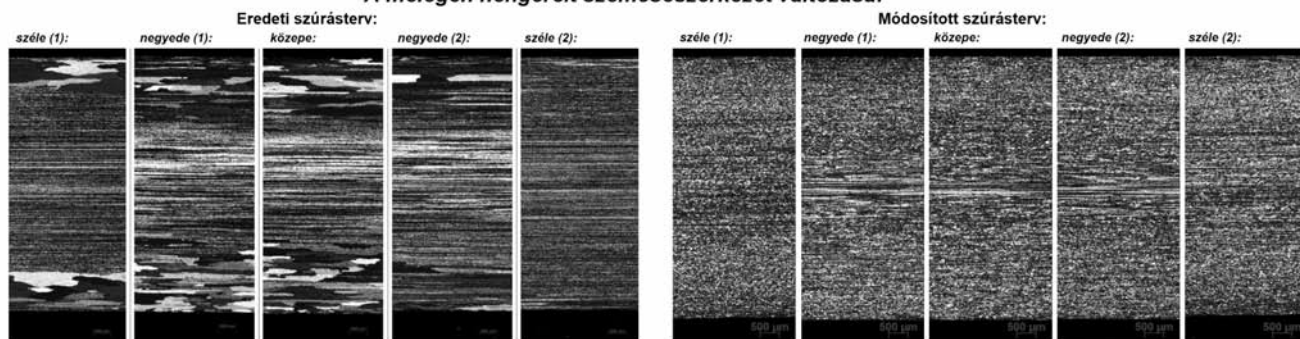
■ 12. ábra. A meleghengерlés fémтani folyamatainak fizikai szimulációja, és az ennek eredményei alapján módosított szűrőrásterv hatása a szemcseszerkezetre
