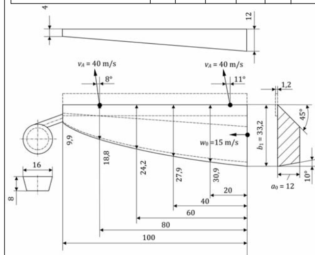
■ 15. ábra. A tangenciális elosztó vázlata és mérettáblázata
