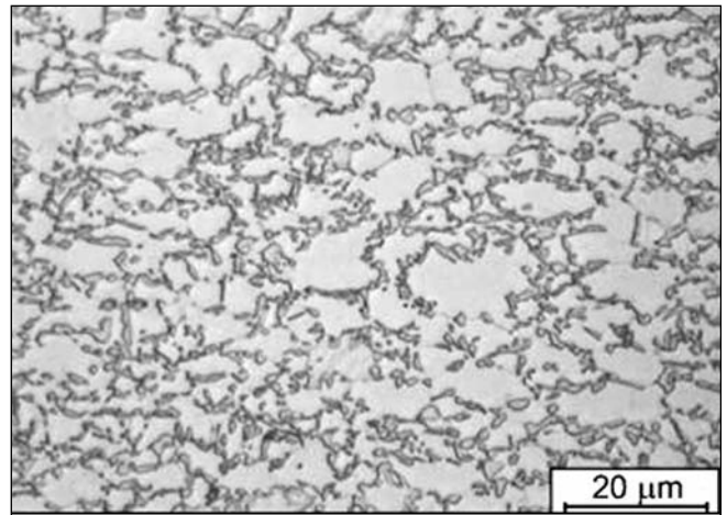
TRIP 690 acél optikai mikroszkópi képe
