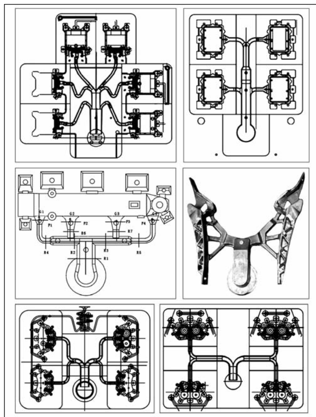
■ 6. ábra. Szűkülő keresztmetszetű elosztórendszer-elágazások az olvadék megfelelő bekötőcsatornákhöz történő elosztásához
