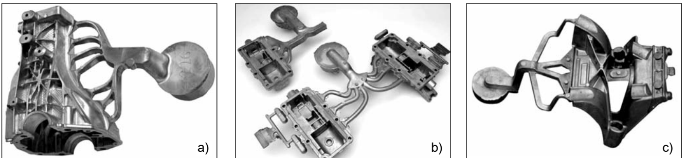
■ 2. ábra. Elosztórendszerek kialakítása több legyező alakú elosztóval nyomásos öntvényekhez a) hátsóhid ház, b) kapcsolófedél, c) vékony falú ház
