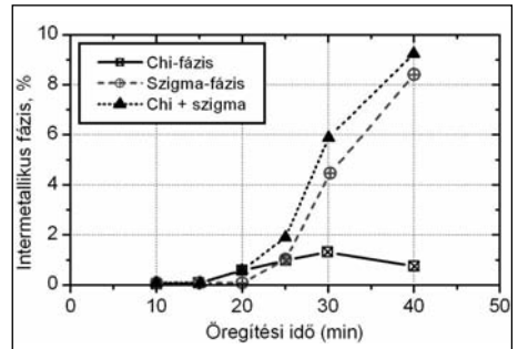
■ 3. ábra. 22Cr-5Ni ötvöztetésű duplex acél 900 °C-on végzett öregítésekor keletkező kiválások képződött mennyisége az öregítési idő függvényében
