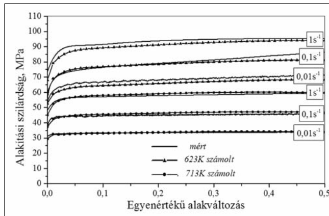
■ 8. ábra. A 713 K-en különböző alakváltozási sebesség esetén mért görbék, valamint a matematikai összefüggés segítségével közelített alakítási szilárdságértékek
