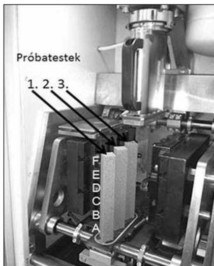
■ 9. ábra. Laboratóriumi maglövőgép a lőtt próbatestekkel
