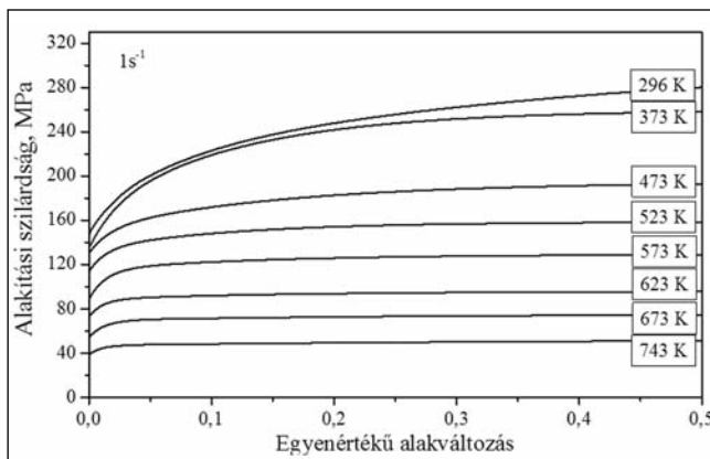
■ 6. ábra. Különböző hőmérsékleten meghatározott alakítási szilárdság-egyenértékű alakváltozás-görbe 1 \text{ s}^{-1} sebességgel zömítés esetén öntött kiinduló állapotú AlMn1 ötvözetben
