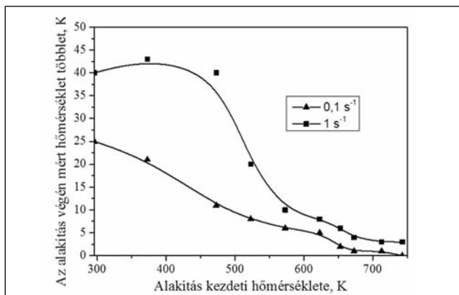
■ 5. ábra. A 0,1 \text{ s}^{-1} és 1 \text{ s}^{-1} alakváltozási sebesség esetén a darabban az alakváltozás végén mért hőmérséklet-többlet az alakítási hőmérséklet függvényében
