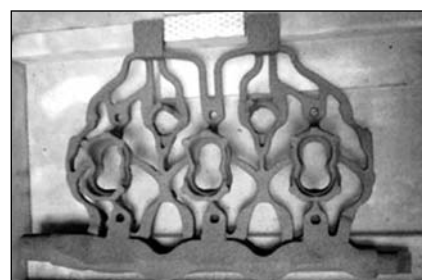
■ 1. ábra. Egy hengerfej üregeinek kialakításához használt bonyolult geometriájú mag
