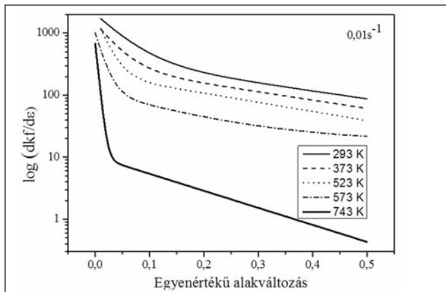
■ 7. ábra. A dkf/d\varepsilon értékei 0,01 \text{ s}^{-1} alakváltozási sebesség esetén különböző alakítási hőmérsékleten az egyenértékű alakváltozás függvényében
