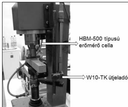
■ 4. ábra. Útjeladóval és erőmérő cellával felszerelt szilárdságvizsgáló berendezés
