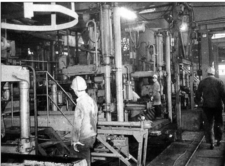
■ 3. ábra. Formázógépsor, 1970
