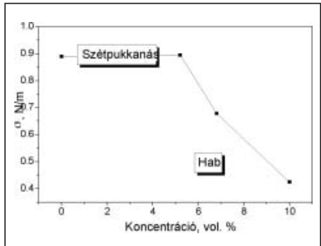
5. ábra. Alumíniumolvadék látszólagos felületi feszültsége az Al_2O_3 -részecské függvényében 700^\circ C -on
