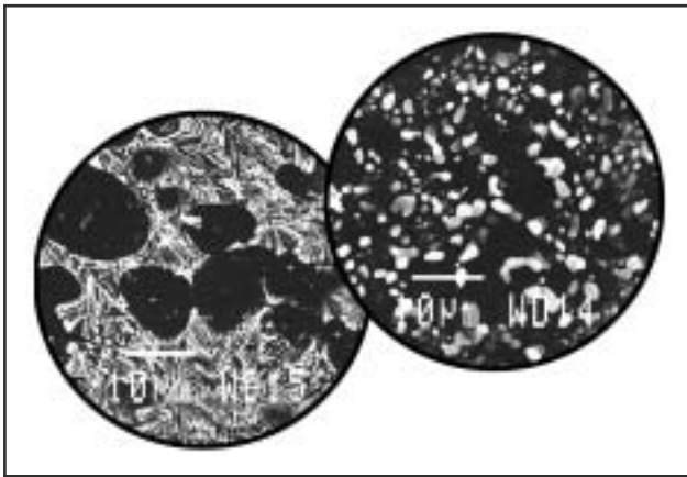
5. ábra. A torzulások alakulása a B-oszlop példáján. Balra AURALTHERM® szerint, levegőn való lehűtéssel, jobbra 490 °C-on, 1 órán át való izzítás, vízben való edzéssel végzett hőkezelés után
