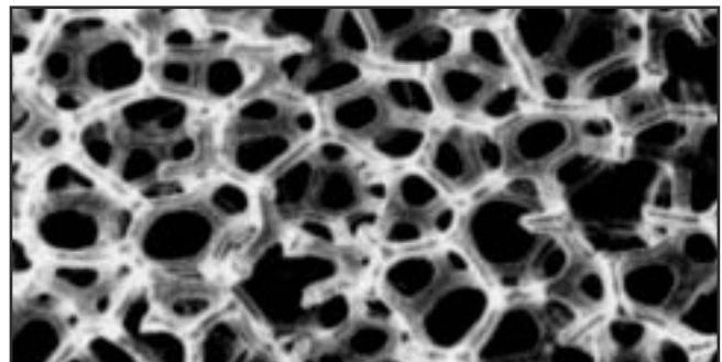
A Duocel® SiC-mátrixú fémhab vázát közel kör keresztmetszetű ágak („ligament”) alkotják. Minden ág finomszemcsés béta-SiC. A Duocel® fémhab széles cella-mérettartományban gyártható: 10-100 PPI (1 PPI = 1 pórus per inch); forrás: http://ergaerospace.com/sic.htm
