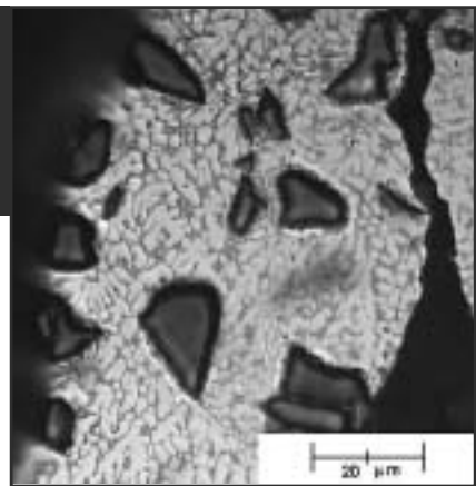
6. ábra. SiC-részecskék felületi szegregációja, gyorsított minta cellafalában (keresztmetszet)
