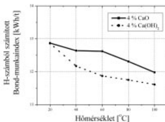
11. ábra: CaO és Ca(OH) 2 diaszporos görög bauxit őrölhetőségére gyakorolt hatása
