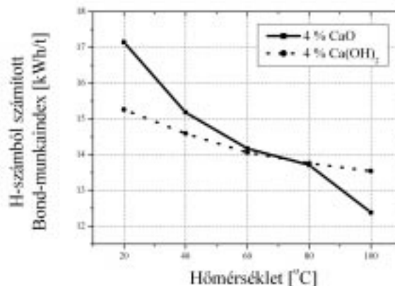
10. ábra: CaO és Ca(OH) 2 böhmtes görög bauxit őrölhetőségére gyakorolt hatása
