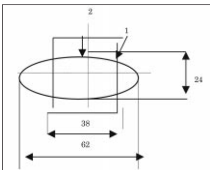
■ 4. ábra. Négyzet-ovál üregpár
