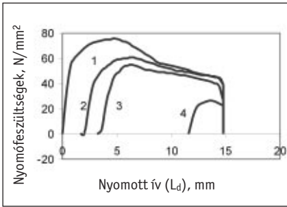
■ 8. ábra. Mért feszültségek a méréspontokban
