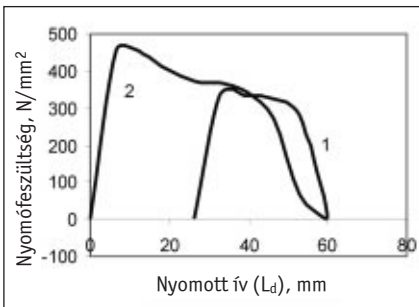
■ 2. ábra. Mért feszültségek a mérőpontokon
