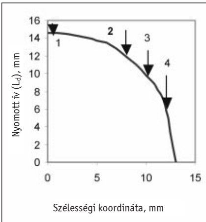
■ 9. ábra. A rúd nyomott felülete a körüregben
