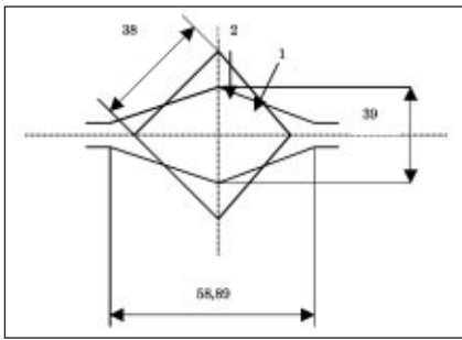
■ 1. ábra. Négyzet-rauta üregpár
