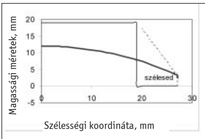
■ 10. ábra. A szélesedés hatása a nyomott felületre
