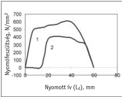
■ 5. ábra. Mért feszültségek a mérési pontokon
