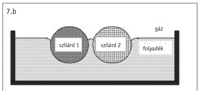
■ 7. ábra. A határfelületi meniszkusz erő definíciójához (a görbült meniszkuszt az egyszerűség kedvéért csak a részecskék mentén jelöltem, valójában azonban az esetek többségében a falak mentén sem vízszintes a meniszkusz)
