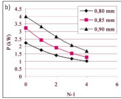
■ 6. ábra. Adott mélységű zóna előállításához szükséges teljesítmény; a) 300 mm/perc, b) 600/mm/perc, c) 900 mm/perc
