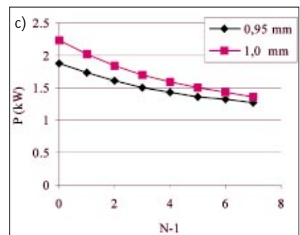
■ 8. ábra. Adott mélységű zóna előállításához szükséges teljesítmény; a) 1500 mm/perc, b) 1800/mm/perc, c) 2100 mm/perc
