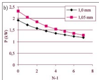
■ 8. ábra. Adott mélységű zóna előállításához szükséges teljesítmény; a) 1500 mm/perc, b) 1800/mm/perc, c) 2100 mm/perc
