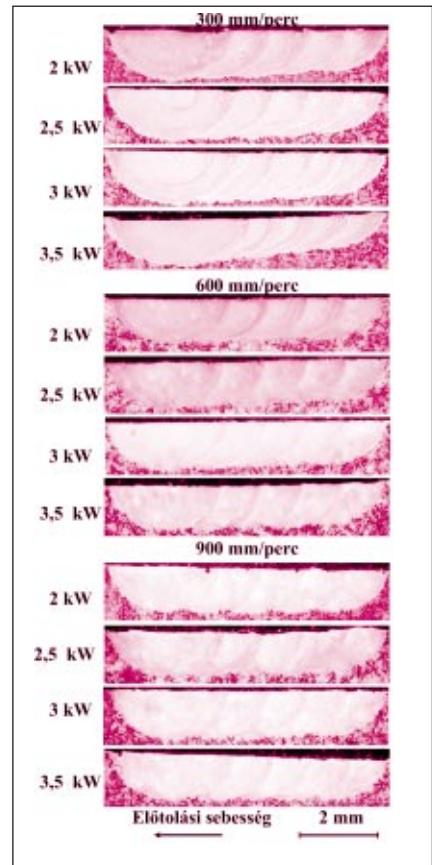
1. ábra. Al7Si10Bi monotektikus ötvözet felületi rétege
