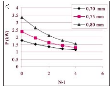
■ 6. ábra. Adott mélységű zóna előállításához szükséges teljesítmény; a) 300 mm/perc, b) 600/mm/perc, c) 900 mm/perc
