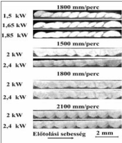
■ 7. ábra. Al-4Cu-1.5Mg-20Pb monotektikus ötvözetek felületi rétegei
