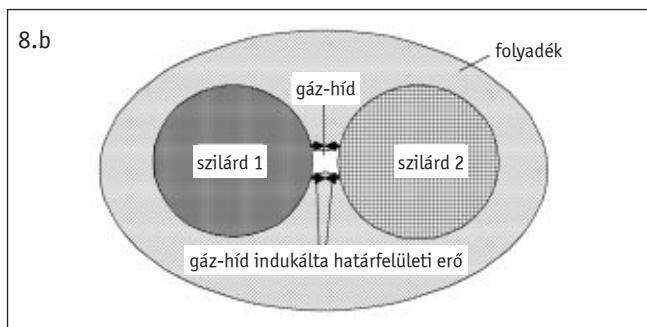
■ 8. ábra. A fluidumhíd által indukált határfelületi erő definíciójához. Folyadék-híd (8.a) és gáz-híd (8.b) által indukált határfelületi erő
