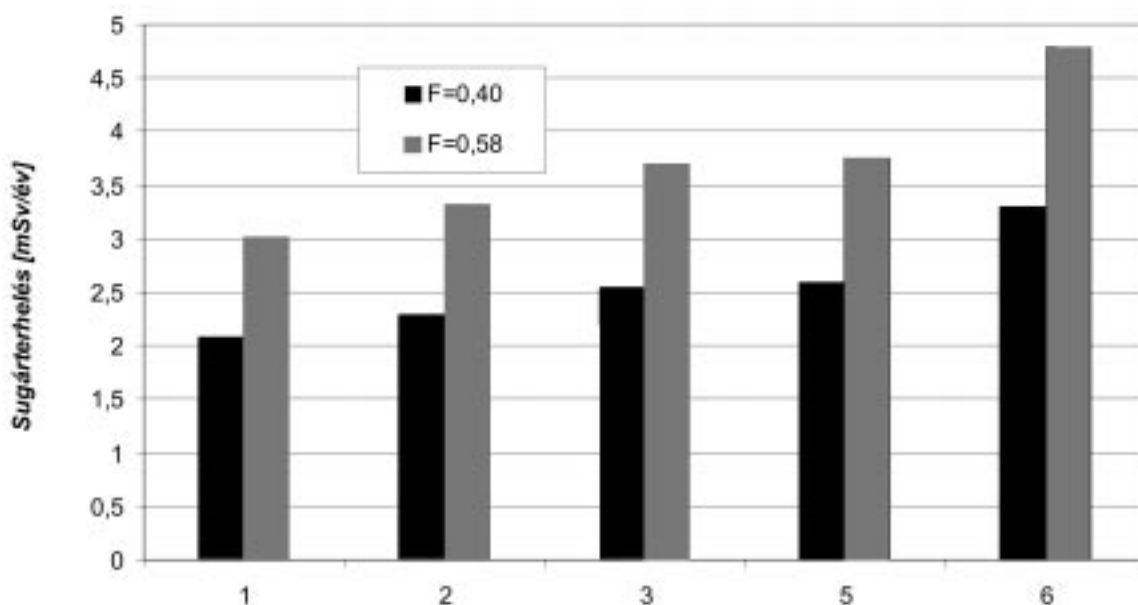
8. ábra: Az ajánlott és a mért egyensúlyi faktorok alapján a föld alatti dolgozók becsült éves sugárterhelése (1, 6: szivattyúkezelő, 2, 3, 5: csapatvezető vājár)
