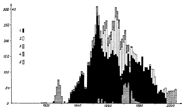
5. ábra Bakonyi mangánércetek termelési diagramja (1917-2003)
