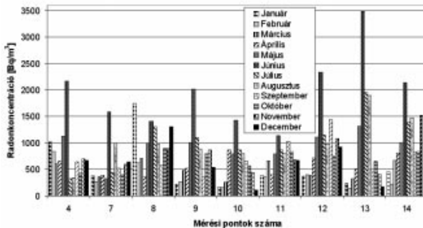
5. ábra: Telepített detektorokkal mért havi átlagos radonkoncentrációk
