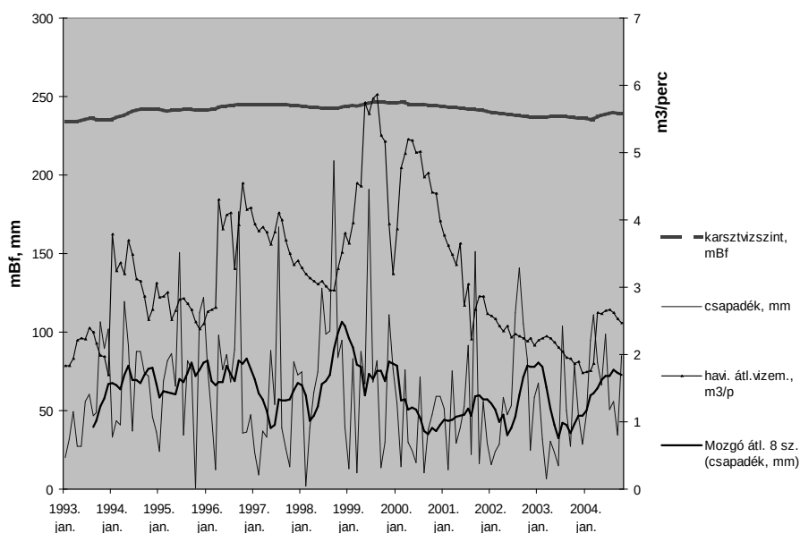
3. ábra: A csapadék, a vízelelés és a karsztvízszint változásai 1993-2004 között
