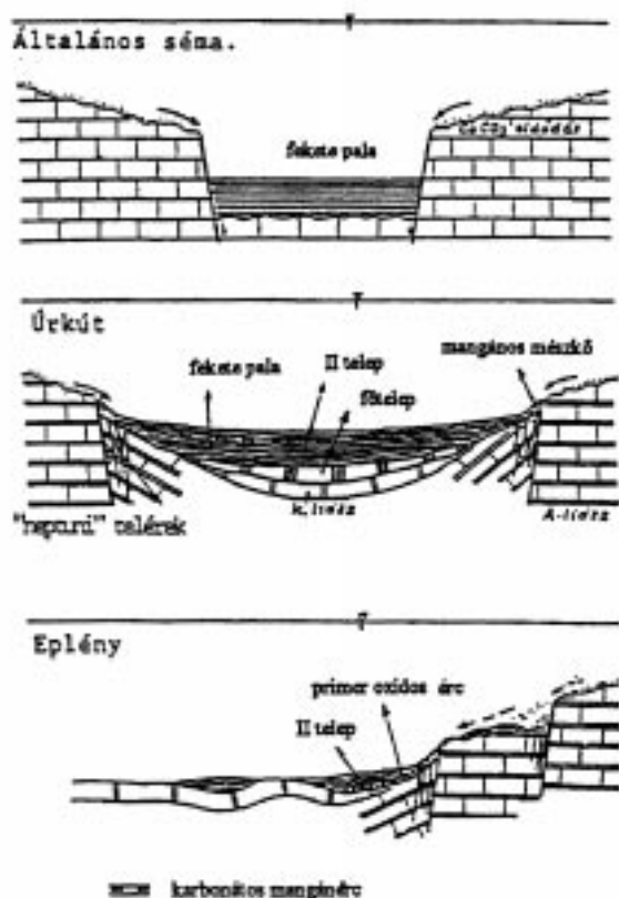
4. ábra Feketepala és diagen karbónátos mangánérc üledékképződési modellje
