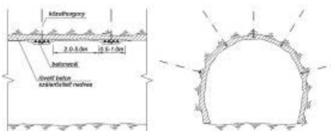
4. ábra: Egy NMT szerint kialakított tipikus szelvény
