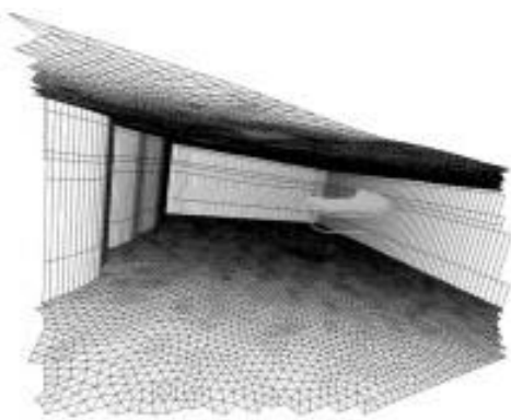
4. ábra: Szivárgáshidraulikai modell: vízkútból indított vízrézecskek útvonala a földtani közegben
