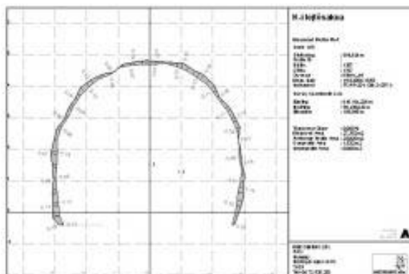
5. ábra: K-i lejtőszakna 598,324 m betonvastagság szelvény
