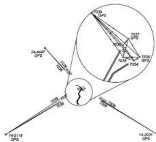
1. ábra: Bátaapáti lejtőszaknak felszíni alappont-hálózata
