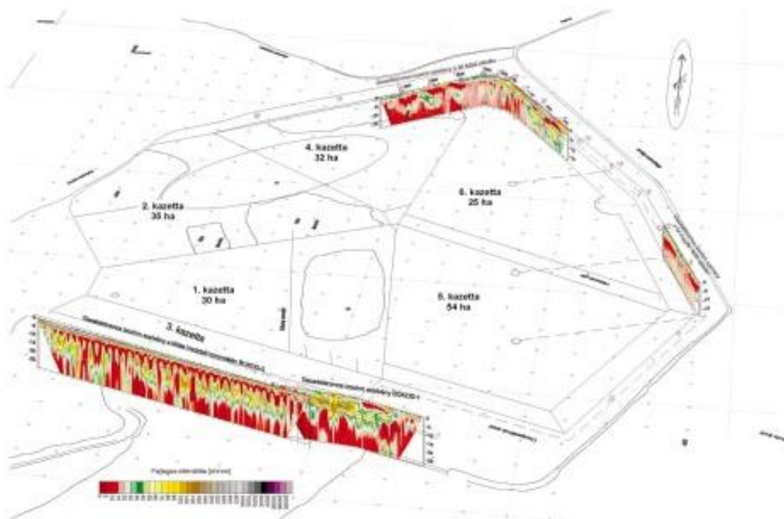
1. ábra: Az oroszlányi zagyvár geofizikai mérései
