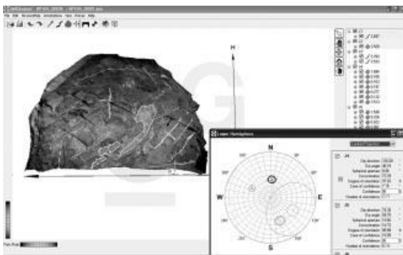
4. ábra: A vágjég 3D-s képe a dokumentált szerkezeti elemekkel és sztereogrammal
