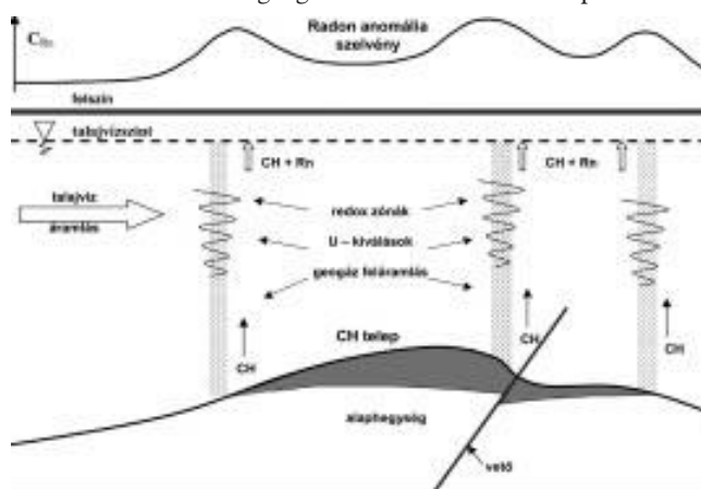
1. ábra: CH-telepek fölött kialakuló radiációs anomália geokémiai modellszelvény-vázlata
