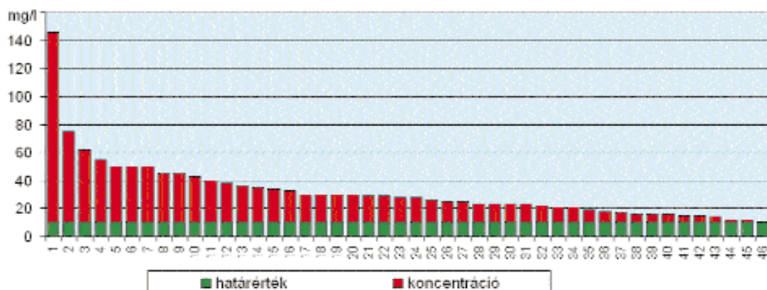
2. ábra: Arzén-előfordulás Csongrád megyében
