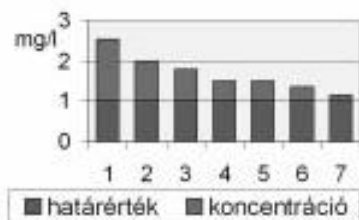
3. ábra: Bór előfordulás a Dél-Alföldön 1: Nagylak, 2: Nagyr, 3: Csanádalberti, 4: Makó-Rákos, 5: Pityvaros, 6: Csanádpalota, 7: Köveg
