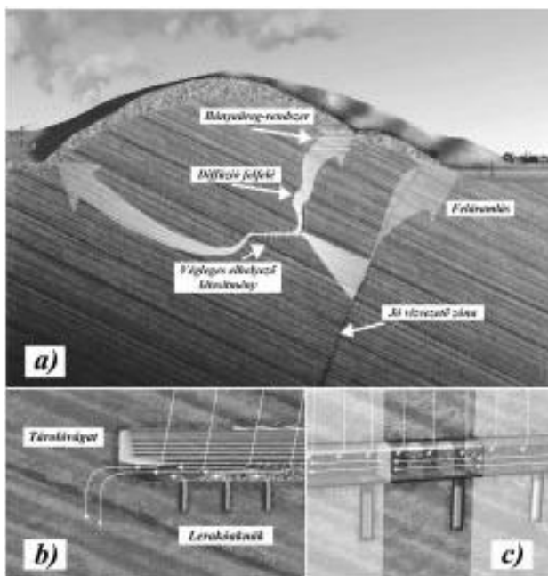
7. ábra: Az egyszerűsített biztonsági értékelés koncepciómodelljének elemei (a: a geoszféra és a bioszféra folyamatai; b: a műszaki gátakban kialakuló áramlási rendszer; c: a tárolóvárat tömedékanyagában kialakuló áramlási rendszer)
