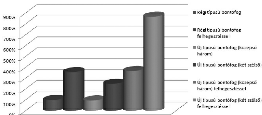
4. ábra: Az új és régi típusú bontófogak élettartamának összehasonlítása
