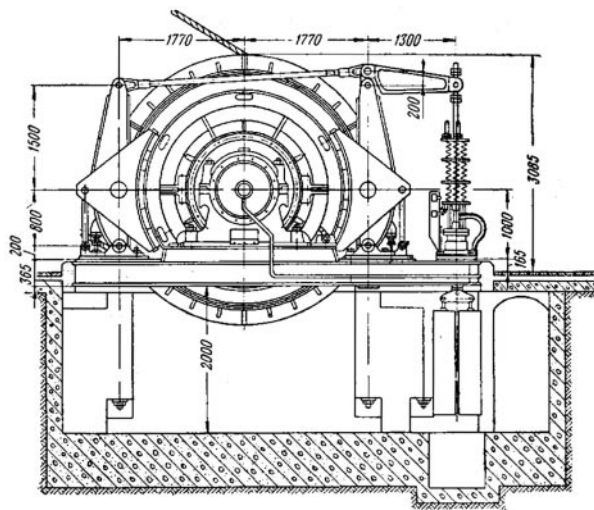
1. kép: A C-3,5X2A típusú egydobos aknaszállító gép alapozási vázlata
