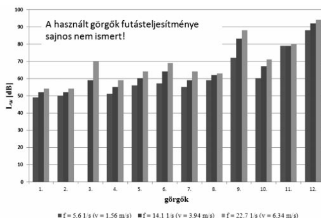
6. ábra: Zajteljesítmény-szintek alakulása új és használt görgők esetén
