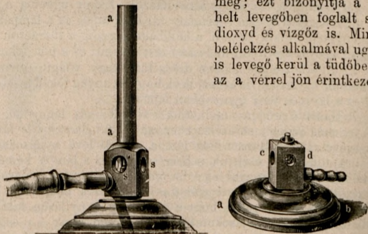
22. ábra. Bunsen-féle lámpa: ab a lámpa alja, cd oldal nyílásai s ezek fölött a gáz kivezető csőve; aa a kémény és balról a gázvezető csőve.
