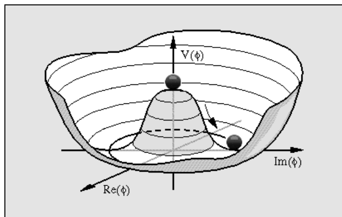
1. ábra: Spontán szimmetriasértés. A Higgs-tér potenciálját ábrázoló sombrero tökéletes hengerszimmetriája elromlik, amikor golyót helyezünk a csúcsára, mert a golyó stabil állapota valahol a völgyben van és legurul, de véletlenszerű, hogy hova esik.
