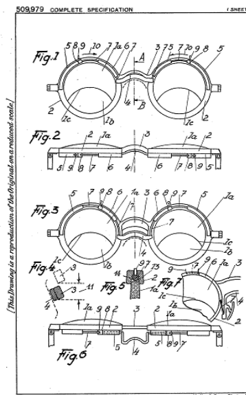
Az elfogadott szabadalmi leírás műszaki rajza 7
