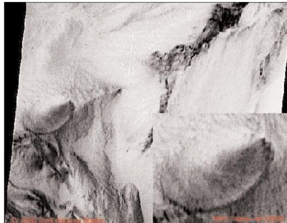
A Mars Global Observer által térképészeti célokkal készített fotószelet egyik részlete. Tisztán látható rajta a „repülő csészealj”. Vajon német? Amerikai? Japán? Netán idegen?
