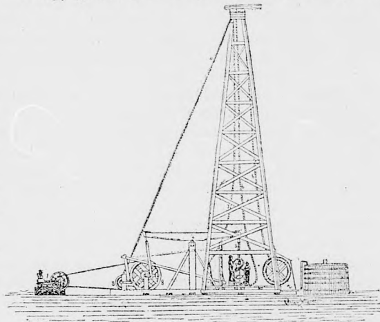
Furási kísérlet gőzerővel.
