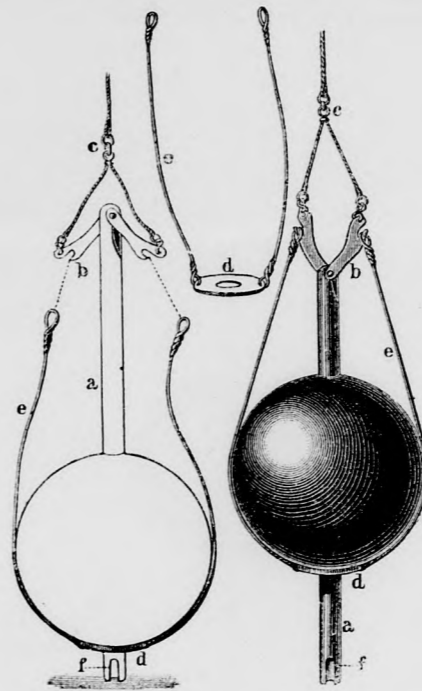
Brooke mélység-mérője.
