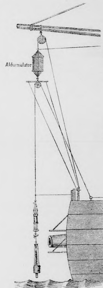
Baillie mélység-mérőjének lebocsátása a tengerbe.
