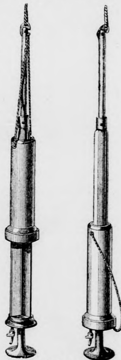
Vizmérő-készülék.
