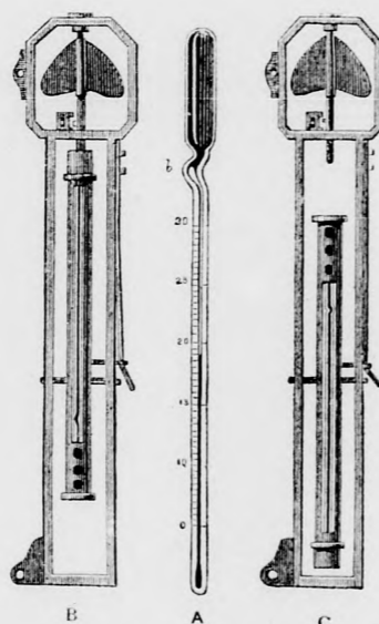
Negretti-Zambra-féle hőmérő.
