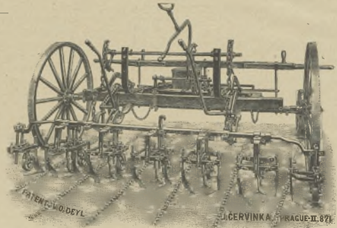
70-ik ábra. A Deyl szabadalmát képező Cservinka-féle kapáló-gép oldalról nézve.
