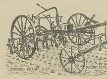
74-ik ábra. A gép beállítva a keresztbe járatott rítkító kapálással.
