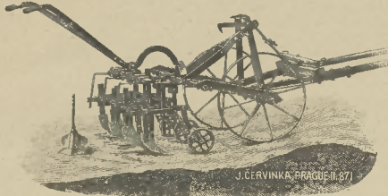
70-ik ábra. A Deyl szabadalmát képező Cservinka-féle kapáló-gép oldalról nézve.
