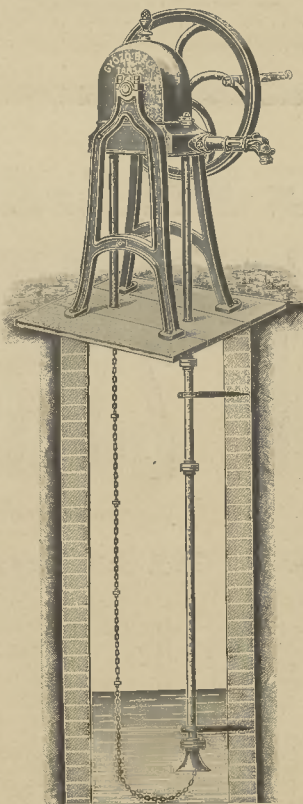
„DIADAL“ láncszivattyu.
