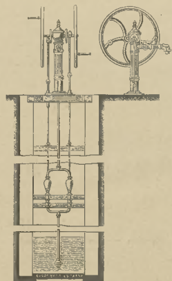
Kéthengerű szivattyu.
