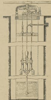
Járgányos szivattyu.
