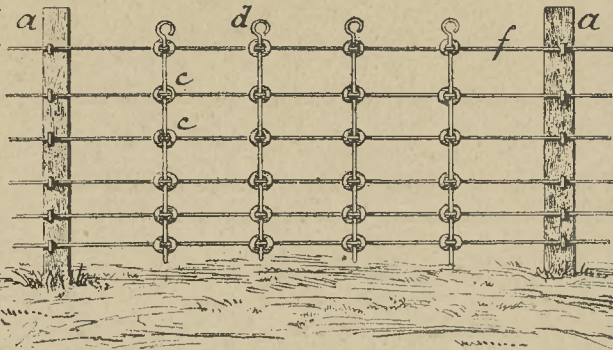
1-ső ábra. Kész amerikai drótkerítés.
