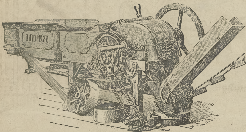
„Ohio“ eredeti amerikai tengeriszártépőgép egyszersmind zöldtakarmányapritó- és szecs-kázó-gép.
