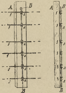
5-ik ábra. A kapcsolás szabályos eszközlésére szolgáló vastag deszkalapok.
