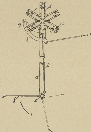
56-ik ábra. A mozgatható gerblyeszerkezet.
