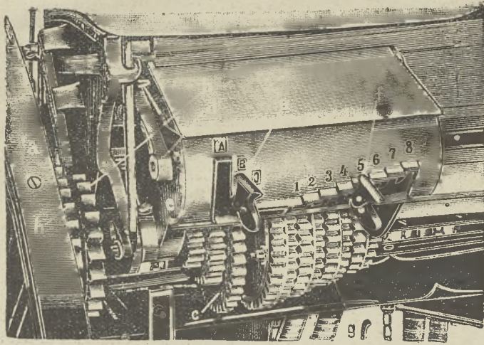
113-ik ábra. A »Saxonia« új mag szabályozója fogaskerek rendszer áttétellel.
