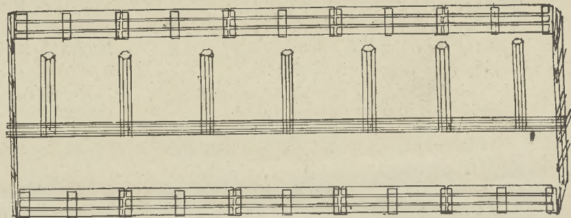
112-ik ábra. 20 méter hosszú, 6 és fél méter széles cukorrépa-prizma szellőztetésének berendezése 1500 métermázsza répa befogadására.
