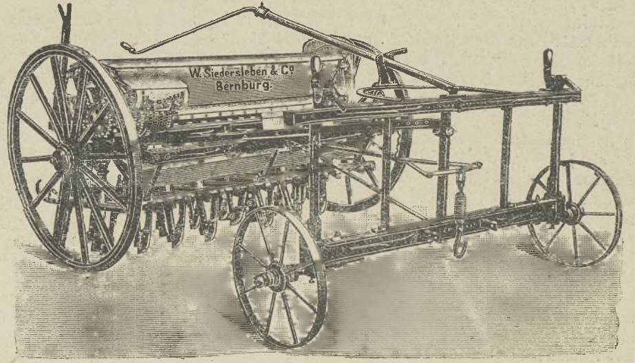
114-ik ábra. A mag szabályozóval felszerelt vetőgép látképe.
