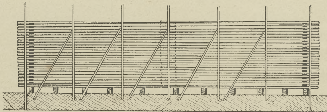
148-ik ábra. Léczgóré oldalról nézve, 6 öl hosszú.
