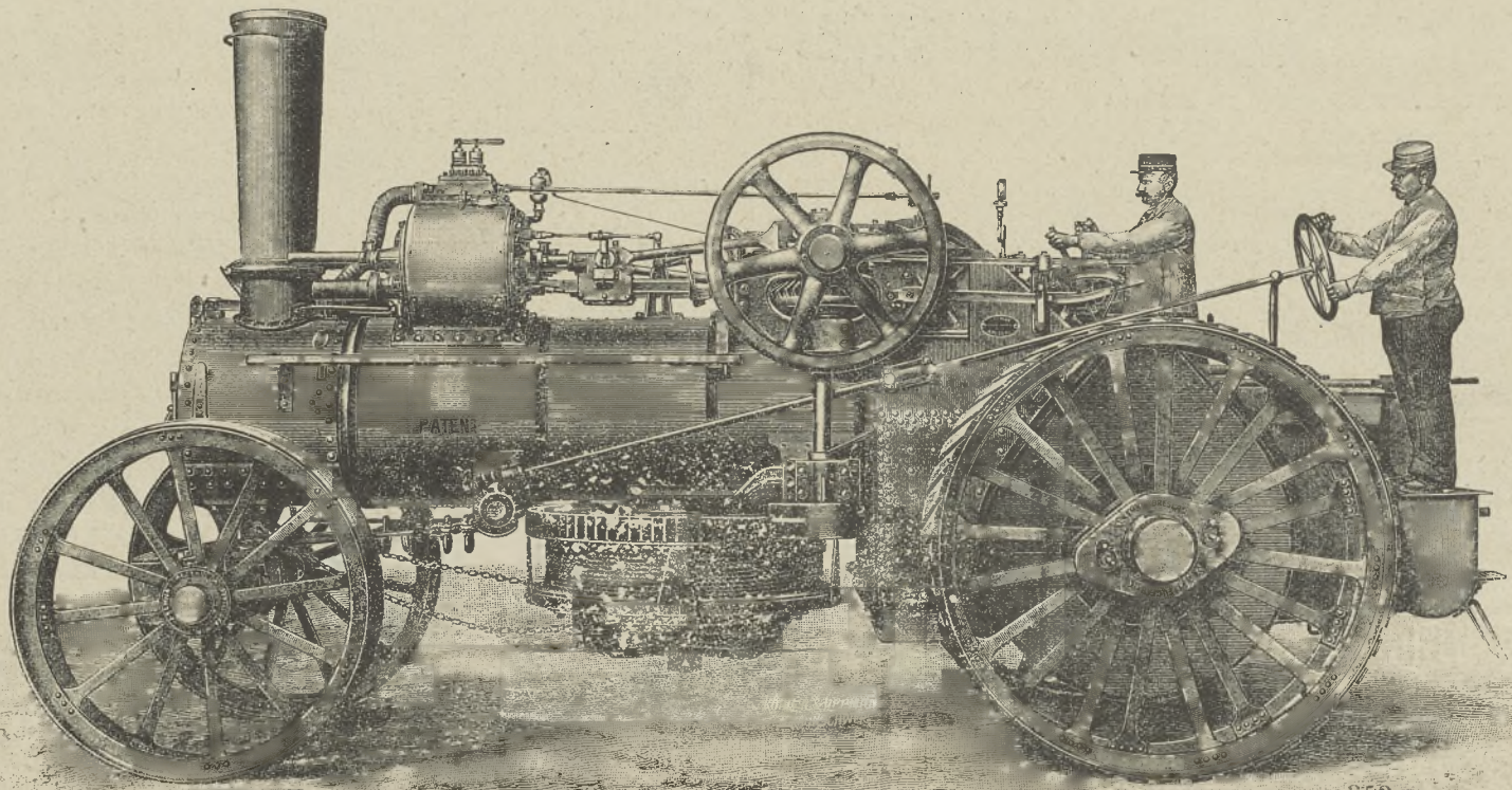
Kemna-féle szabadalmazott forrógőz-ekemozdony oldalnézete.
