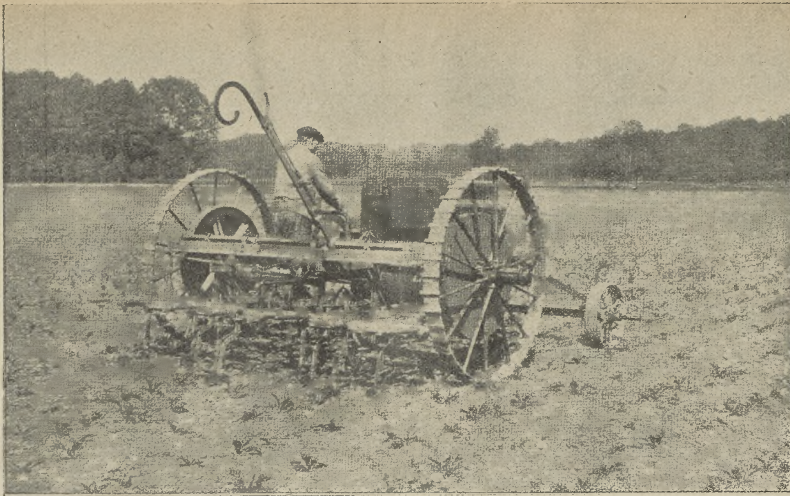
139-ik ábra. Bajac automobilkapája menetközben.
