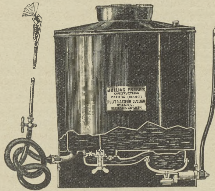
88-ik ábra, Jullian Freres permetezője.
