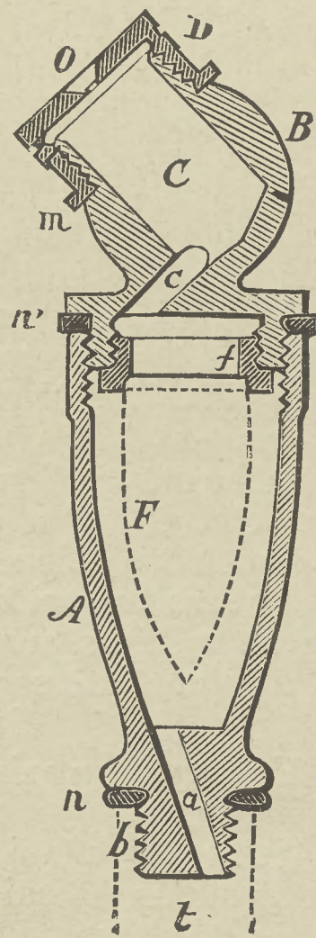
89-ik ábra. A szóró szerkezet.
