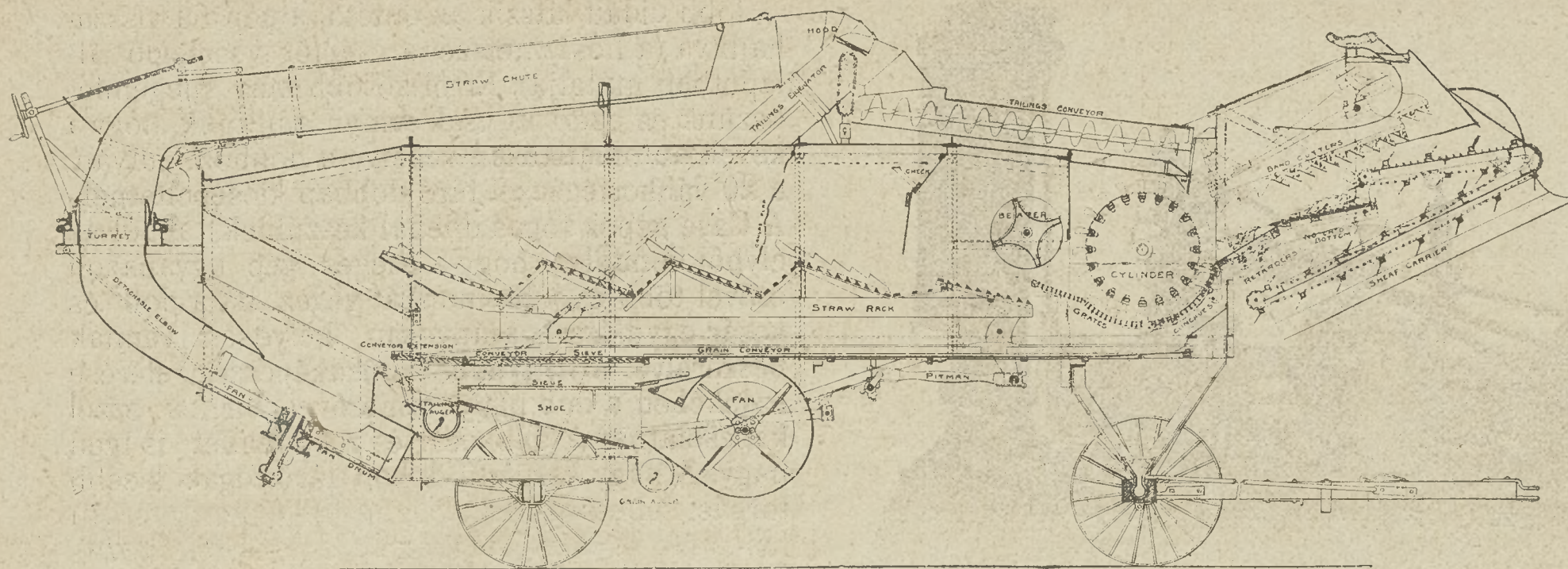
91-ik ábra. »Case« automatikus cséplő hosszmetsete.
