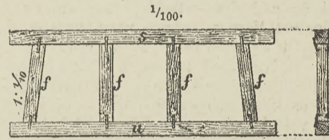
113-ik ábra. Faragott fából (gerendákból) készült hidbak.
