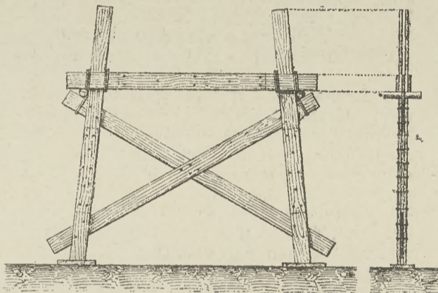
112-ik ábra. Gömbölyű fából (fenyő) készült hidbak.
