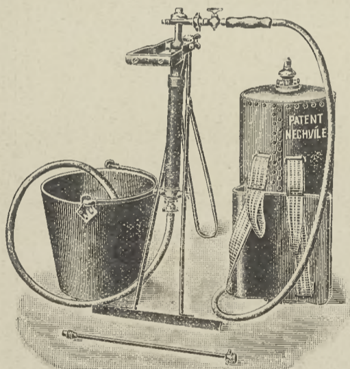
„Automata“ önműködő-fecskendő öltető szivattyúval.
