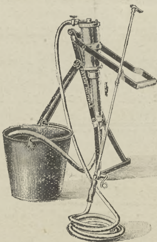
„UNIKUM 2“ „Unikum“ mázó- és fertőtlenítő fecskendő a cs. és kir. hadseregnek, mint legjobb módszerü, be van vezetve, megakadályozza a ragályos betegségek elterjedését, fontos eszköz minden mezőgazda részére.
