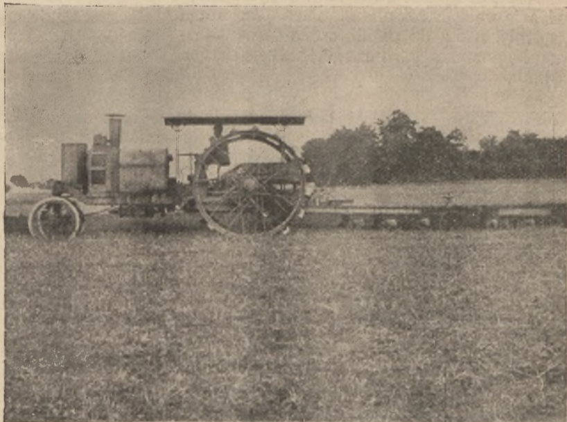
75-ik ábra. Wiss Süddeutsche Ind. Ges. benzin traktorja.
