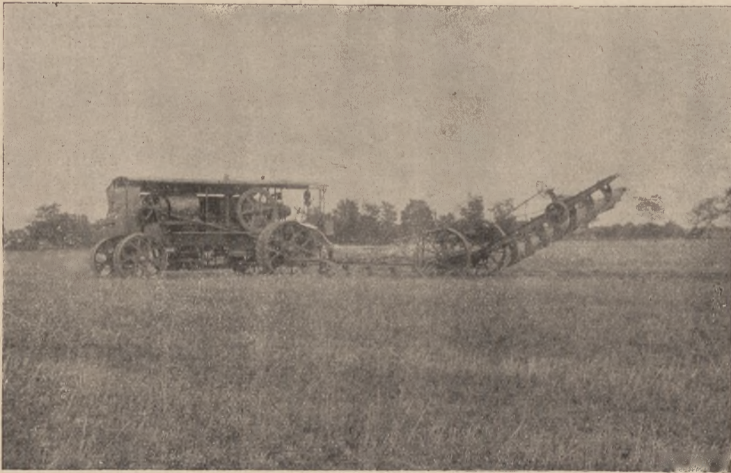
84-ik ábra. Gibás nyersolajmotoros két géprendszerű eke.
