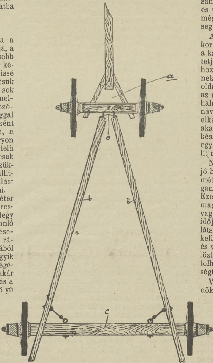
26-ik ábra. A vontató masina vázlata.
