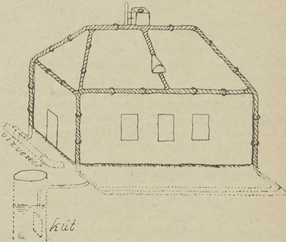
44-ik ábra. Findeisen tanai szerint berendezett villámhárító szerkezet.
