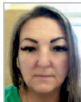
Bordás Judit
