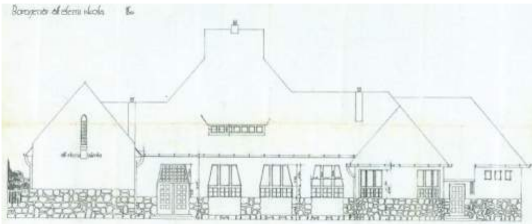
Tervezett főhomlokzat
