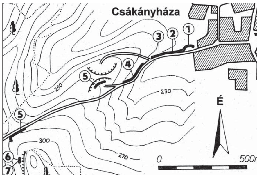
A csákányházi földtani szelvény vázlatos térképe. Jelmagyarázat: 1. tengeri homokkő a felhagyott homokbányában, 2. ferde rétegzettségű homokkő, 3. kőzetliszt apró kagylókkal (Csákányházi Tagozat), 4. átmenet a szárazföldi üledékekbe, 5. folyóvízi kavics és homok, feljebb agyagrétegekkel, 6. beomlott táró, 7. riolituffa szénréteggel • Gaál Lajos rajza
