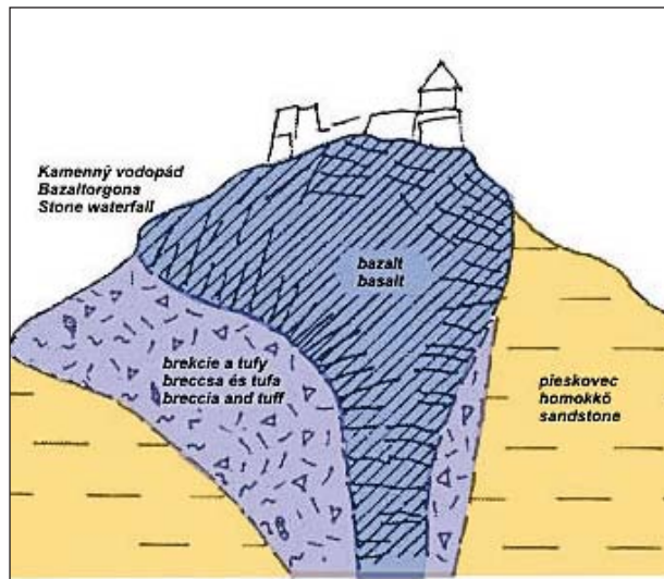
A somoskői várhegy földtani metszete (Konečný 2004 nyomán)
