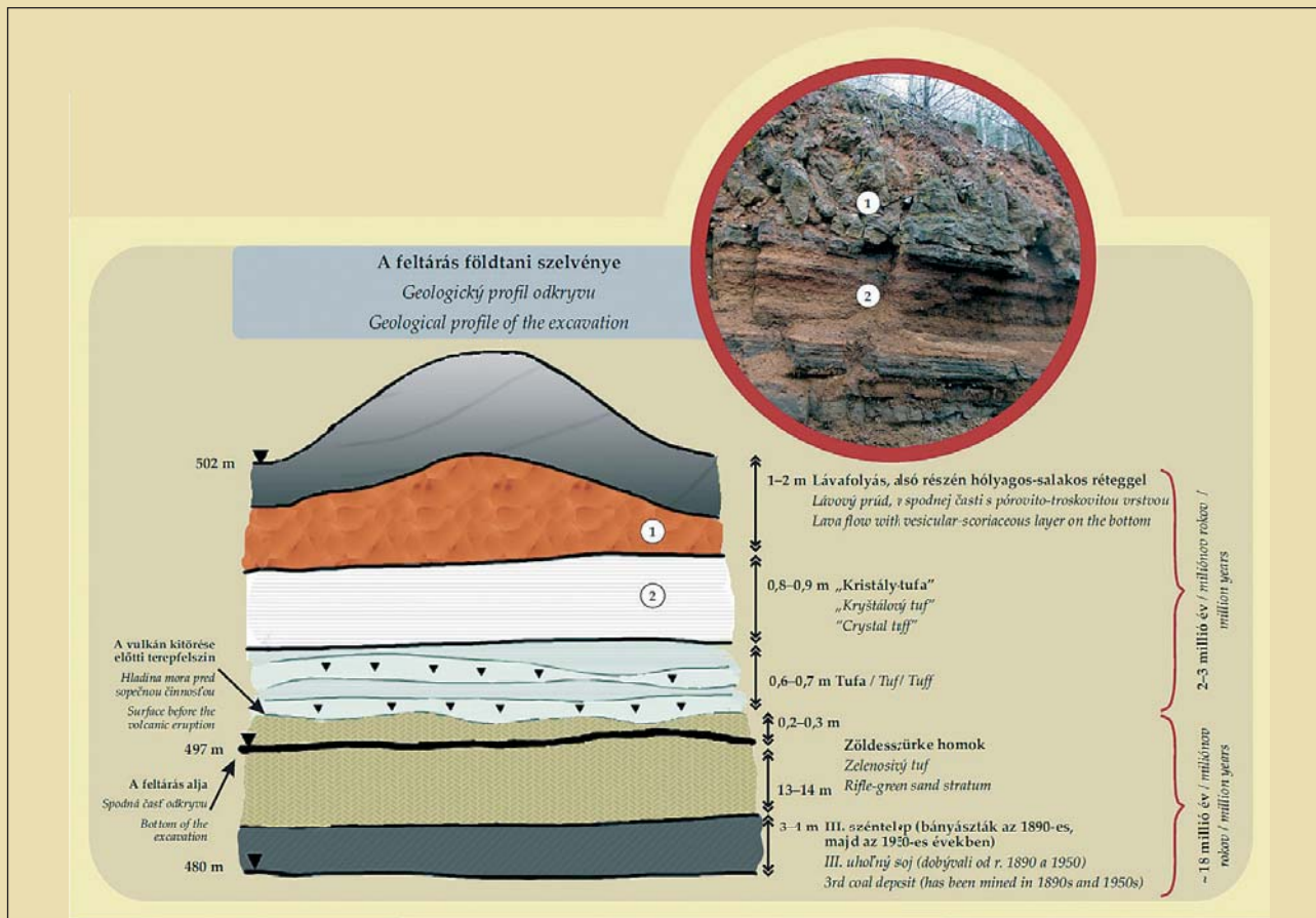
Az Eresztvényi kőbánya évmilliókat átölelő feltárása
