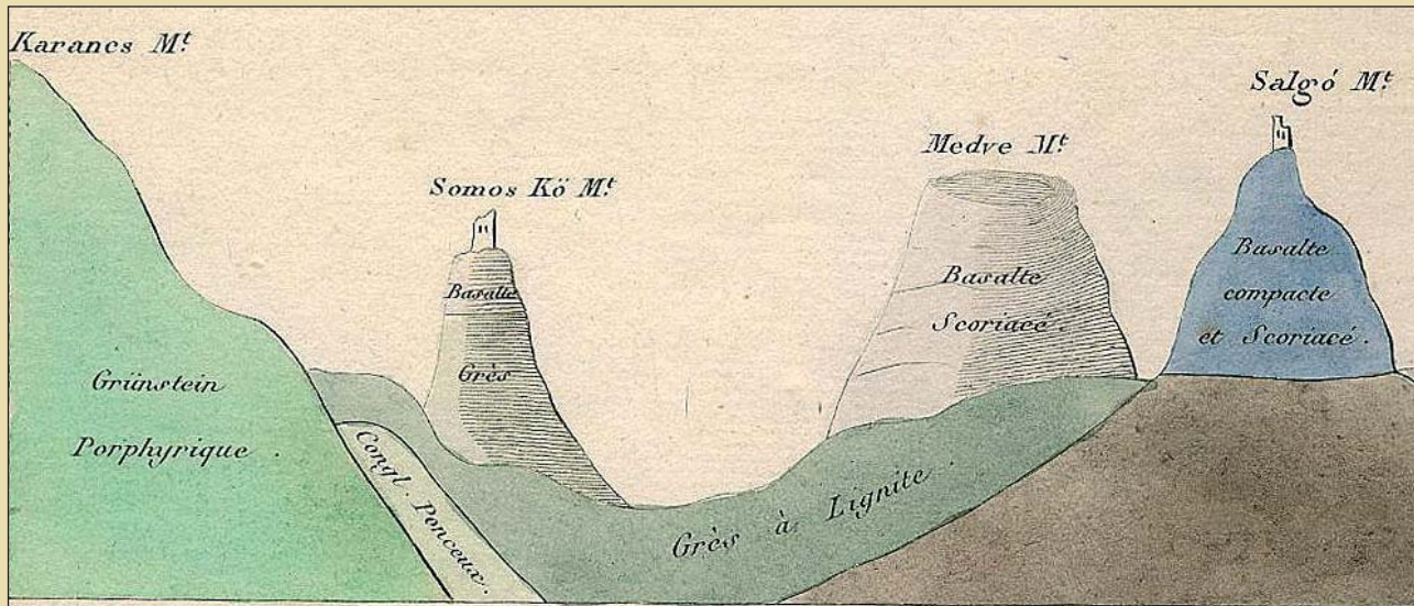
Beudant földtani szelvénye a Karancstól a Medvesen keresztül a Salgóig, 1818-ból
