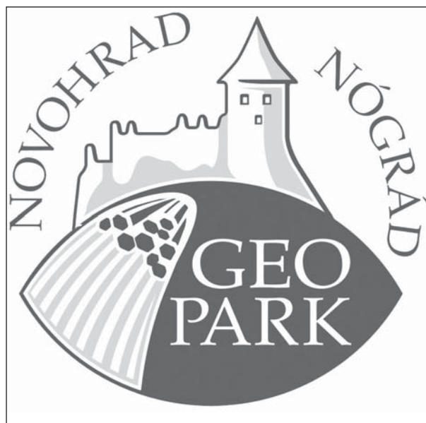
A somoskői hajlott bazaltszlopok a Novohrad-Nógrád Geopark logójában
