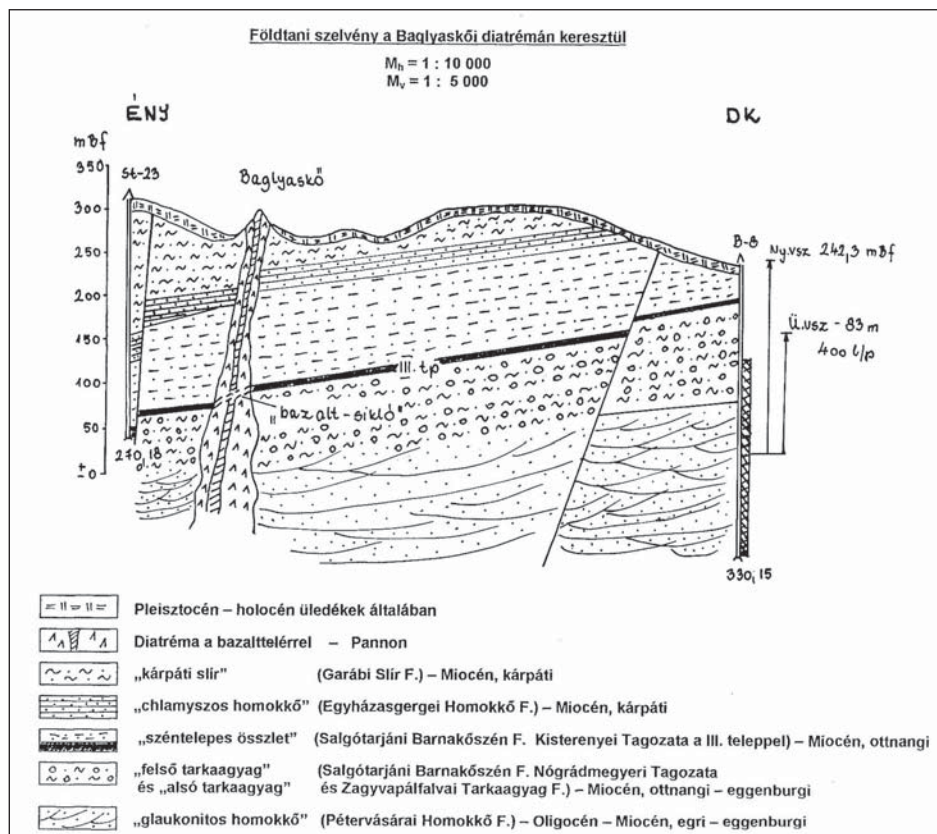
Baglyaskő - földtani szelvény • Prakfalvi Péter rajza
