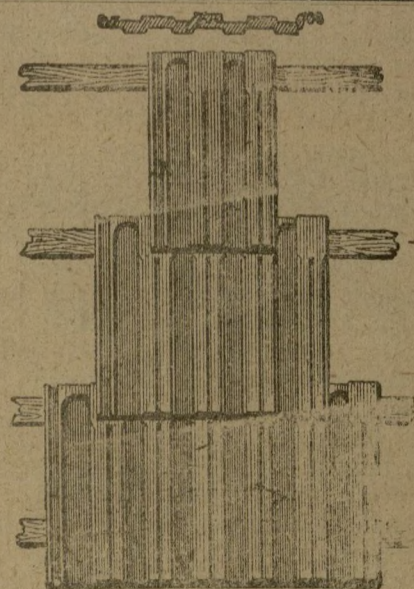
Zombolyai gyártmány Szab. biztonsági préselt átfedő cserép 253. szám.
