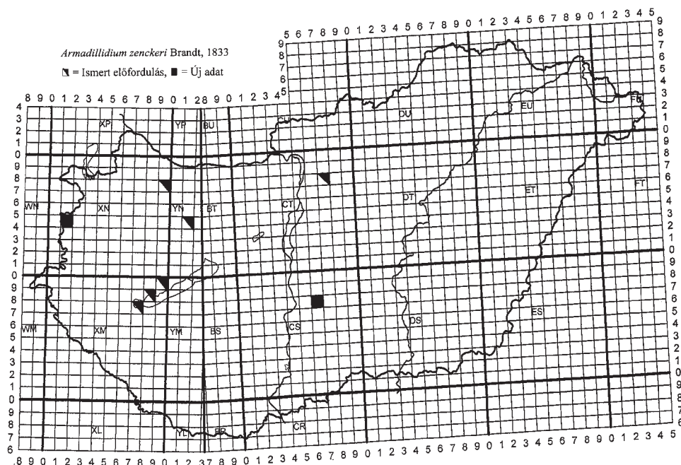
6. ábra: Az A. zenckeri előfordulása Magyarországon
