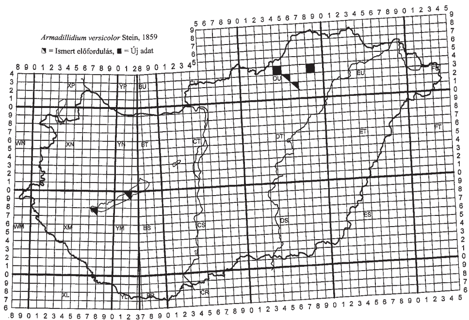
5. ábra: Az A. versicolor előfordulása Magyarországon
