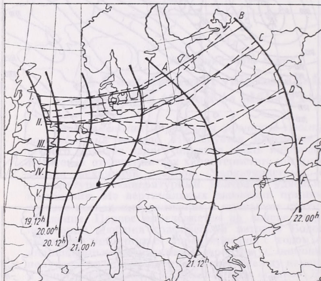
3. ábra: A hideg front helyzete és trajektóriái 1959. január 19-én és január 22-én 00h között. A római számmal jelzett trajektóriák (vékony vonalak) konvencionálisak, a betűkkeljelzett trajektóriák (szaggatott vonalak) a front normálisának irányával egyeznek meg
