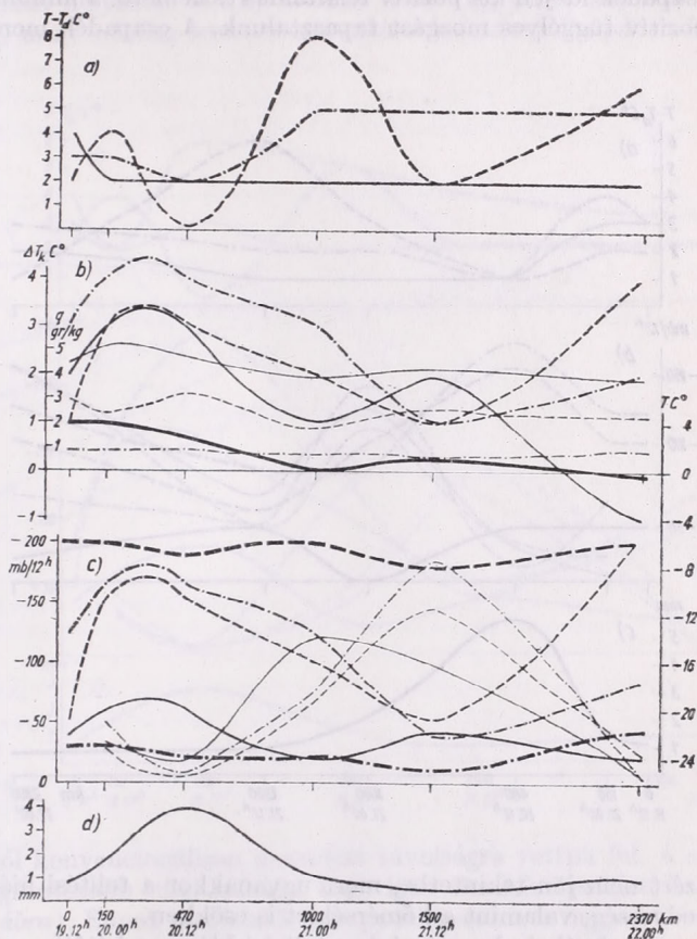
4. ábra: A front szerkezetét jellemző karakterisztikák eloszlása a hideg front C trajektóriája mentén: a) A telítési hiány eloszlása; a folytonos vonal a 850, a szaggatott vonala 700, a pontozott szaggatott vonal az 500 mb-os felületre vonatkozó értékeket jelöli. b) A specifikus nedvesség (vékony vonalak); a hőmérsékleti kontraszt (középvastag vonalak); és a hőmérséklet (vastag vonalak) eloszlása. Az egyes szintek jelölése megegyezik a)-val. c) A vergenciális (vékony vonalak) és a frontális (középvastag vonalak) függőleges sebesség eloszlása mb/12 órában. A negatív értékeket a szemléletesség kedvéért vettük pozitív irányban. d) A csapadék mennyiségének eloszlása mm-ben
