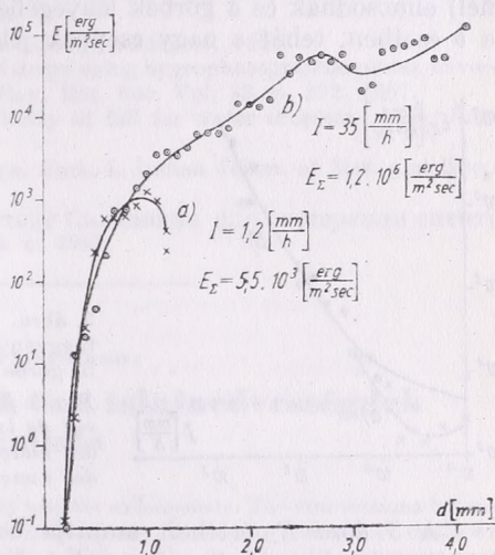
2. ábra. Az esőcsepp-erózió eloszlása két individuális esetben az átmérő függvényében: a. görbe: folytonos eső (1959. XII. 7. 12 h 27'), b. görbe: záporosó (1960. VII. 21. 12 h 03')
