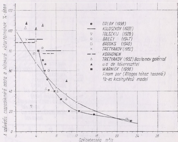
3. ábra. A szilárd gallérral védett csapadékmérőben mért hó és a közvetlen környezet hótakarója víztartalmának viszonya különböző szélsébségeknél
