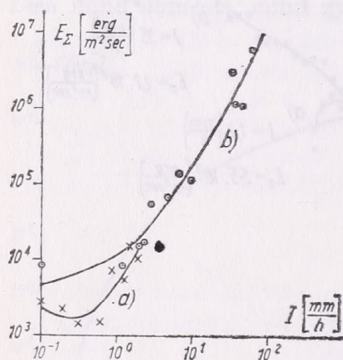
3. ábra. Az esőcseppek eróziója a csapadék-intenzitásának függvényében: a. görbe: réteges felhőkből hulló esőkre, b. görbe: gomolyos felhőkből hulló esőkre
