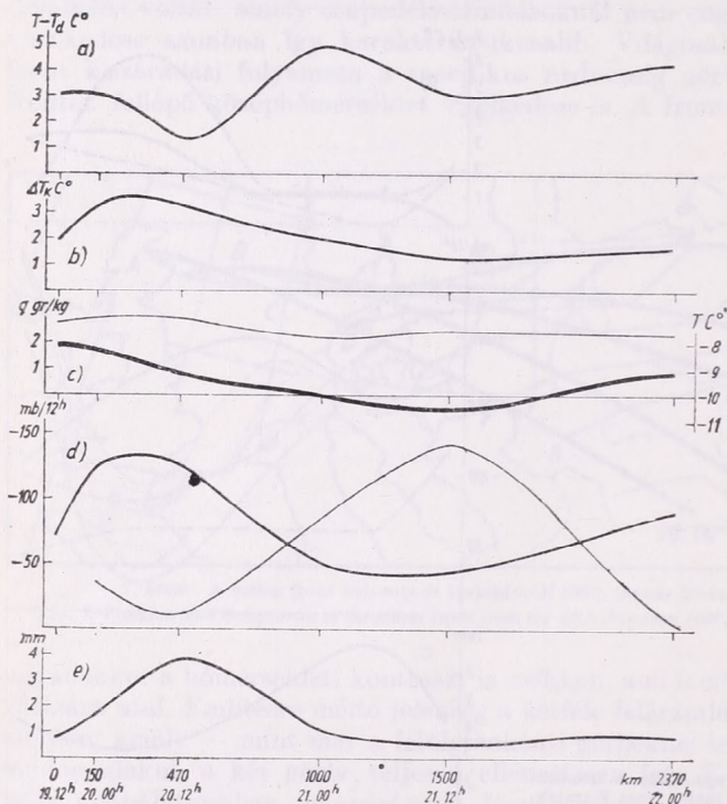
9. ábra: A közepse karakterisztikák eloszlása a hideg front C trajektóriája mentén: a) a telítési hiány; b) a hőmérsékleti kontraszt; c) a specifikus nedvesség és a hőmérséklet; d) a frontális és vergenciális feláramlás; e) a csapadék eloszlása
