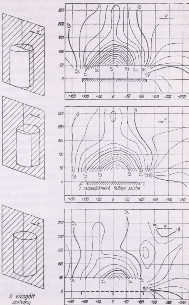
5. ábra. A sebességek alakulása a csapadékmérő edény felett
