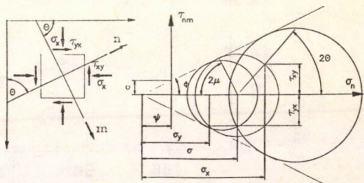
Fig. 3.: Mohr - Coulomb failure
