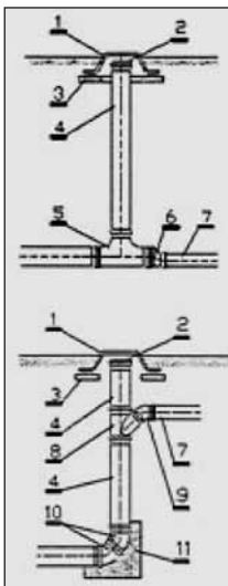
Műanyag csőrendszer
