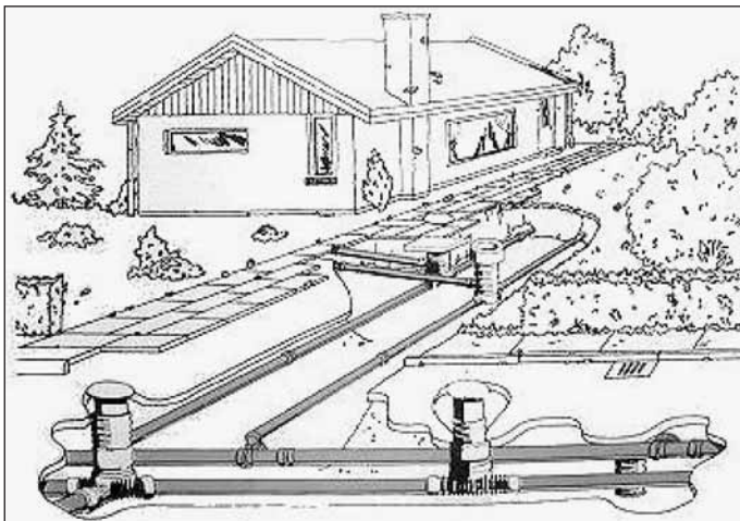
Műanyag csőrendszer
