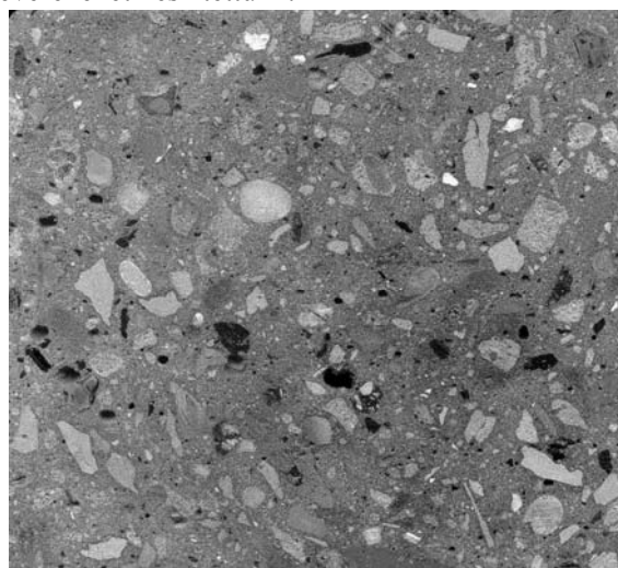
8. ábra Vegyes törmelék adalékanyagú, újrahasonított beton struktúrája
