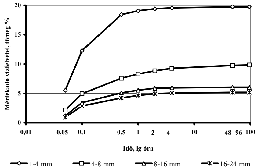
4. ábra Betontörmelék frakciók mértékadó vízfelvétele az idő függvényében
