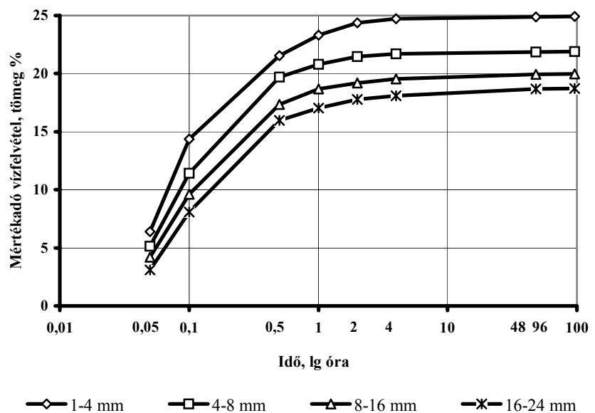
5. ábra Téglatörmelék frakciók mértékadó vízfelvétele az idő függvényében
