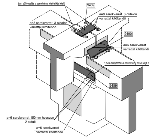
Főtartó – szelemen hegesztett kapcsolata
