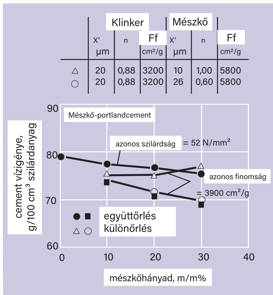
7. ábra: A cement vízigényének változása a mézskőhányad függvényében (együttörlés és különőrlés) [8]
