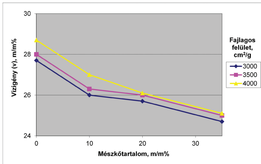
6. ábra: A cement vízigényének (v) változása a mézskőtartalom függvényében (együttörlés)
