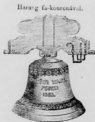
Fakorona régiebb szerkezettű
