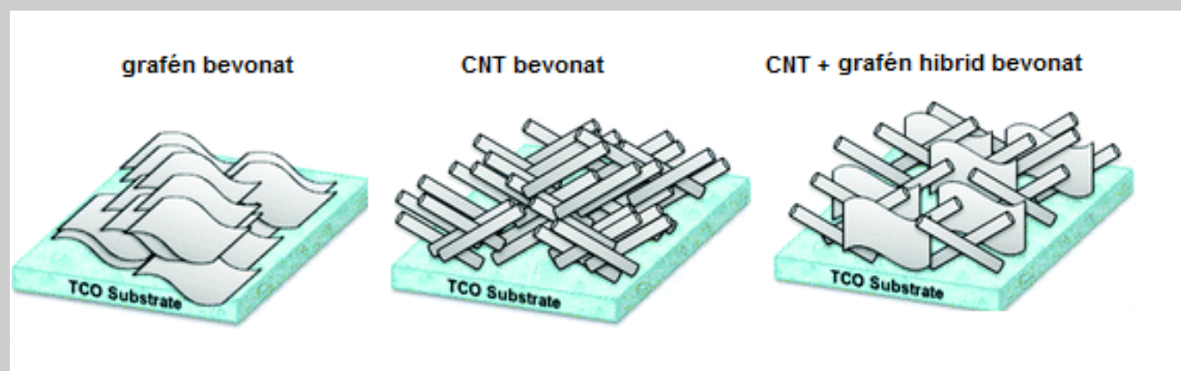
6. ábra. 3D szén allotróp elektromosan vezető bevonatok fotóanód felületen foto-elektrokémiai vízbontó cellában (19). TCO substrate: transparent conducting oxide átlátszó vezető oxid hordozó.
