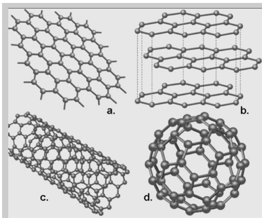
1. ábra. Szén allotrópok sematikus ábrázolása, a: grafén; b: grafit (grafén rétegek egymáson); c: szén nanocső (grafén feltekeredve); d: C 60 , Buckminsterfullerén (grafén felületű, 20 hatszögű és 12 ötszögű lappal határolt poliéder).
