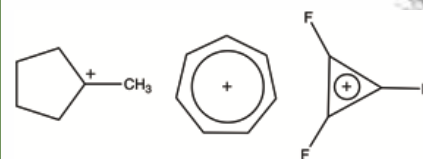
7. ábra Stabilis karbokationok néhány képviselője
