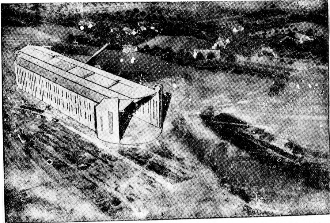
Az új léghajócsarnok Friedrichshafenben. Friedrichshafen-Löwentalban most készült el egy újabb óriási léghajócsarnok, amely teljesen acélból készült. Az új léghajócsarnok 53 méter magas és 58 méter széles.
